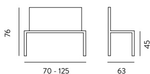
Art. 991/1 Tube poltroncina
